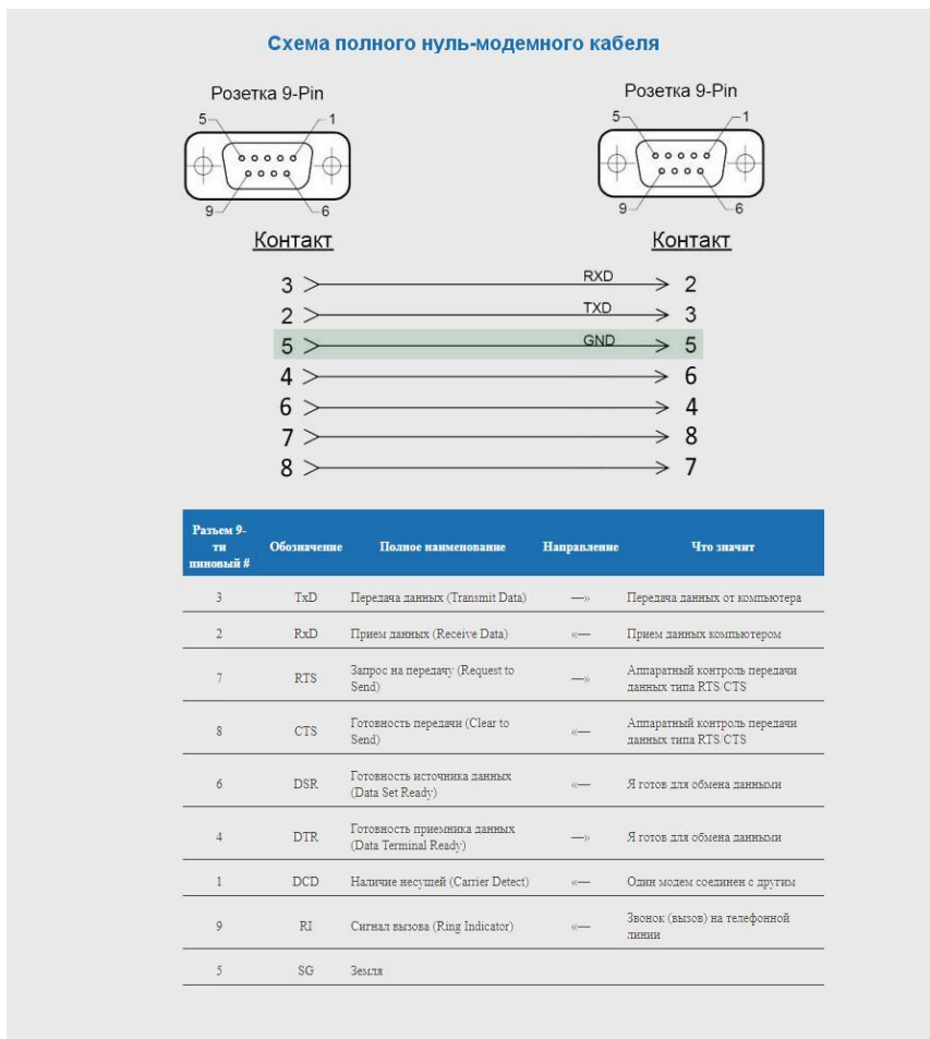
Рис. 25. Схема распыки нуль-модемного кабеля для связи с АТС
