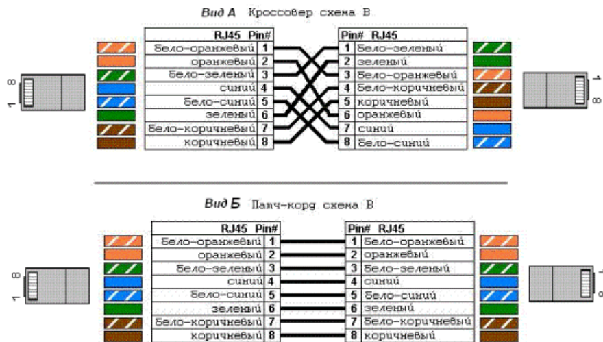
Рис. 26. Схема распылки ETHERNET кабеля для связи с АТС
