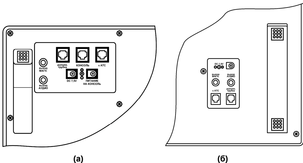
Рис. 3. Разъемы на нижней стороне корпуса пульта РЕГИОН-ЦМП (а) и РЕГИОН-ЦЛП (б).
