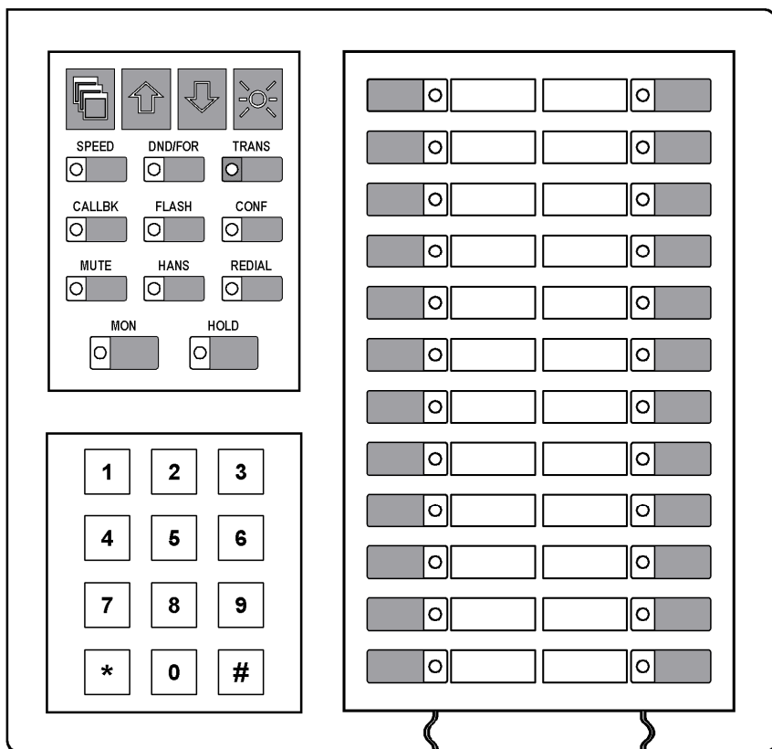
Рис. 6. Расположение клавиш на пульте РЕГИОН-ЦЛП.
