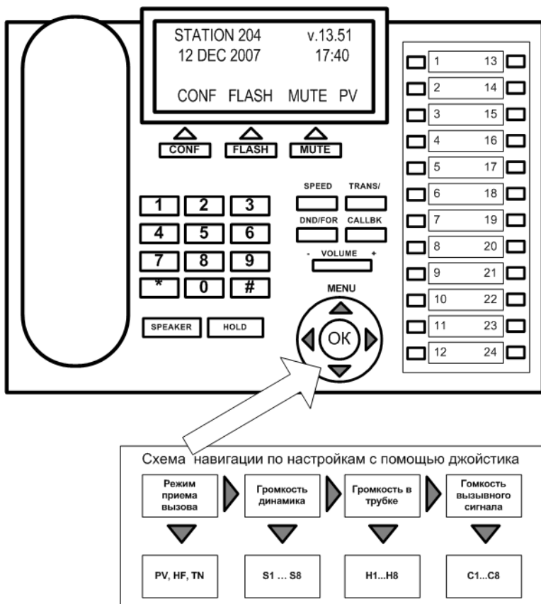
Рис. 1. Расположение клавиш на пульте ALDP-7224D.
