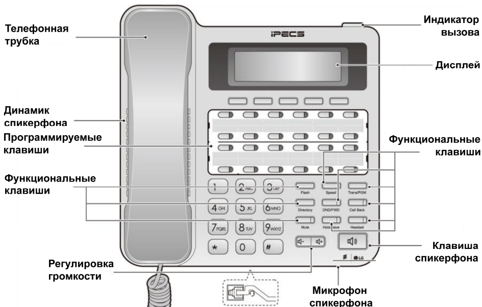
Рис. 1. Внешний вид системного аппарата LDP-9224DF.
