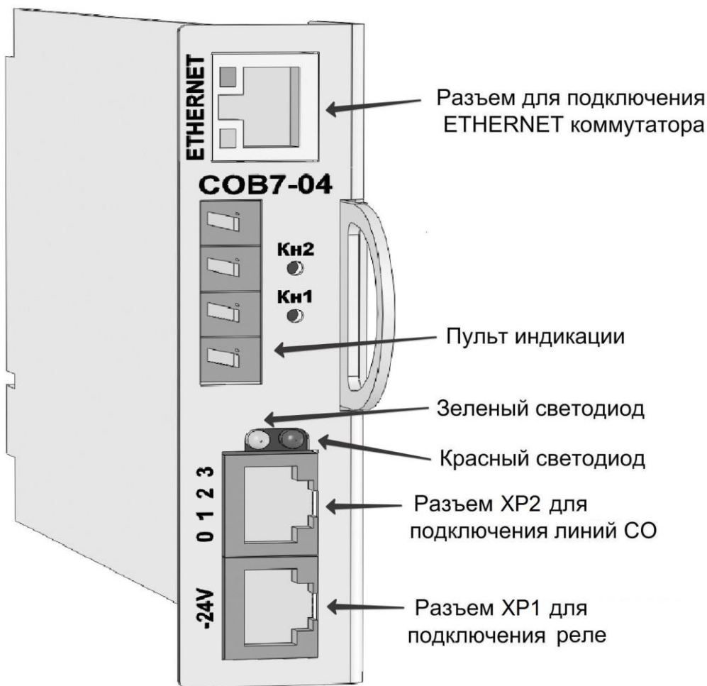
Рис. 5. Модуль COB7-04
