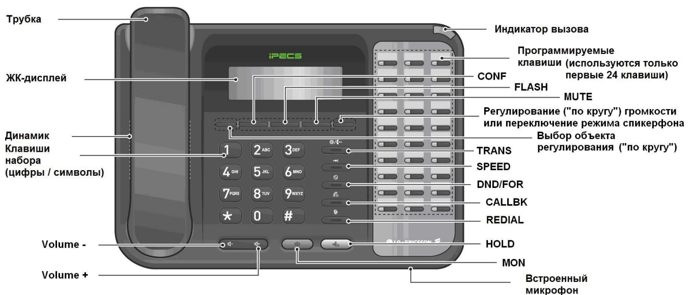
Рис. 6. Расположение клавиш и схема навигации системного аппарата ALDP-9030
