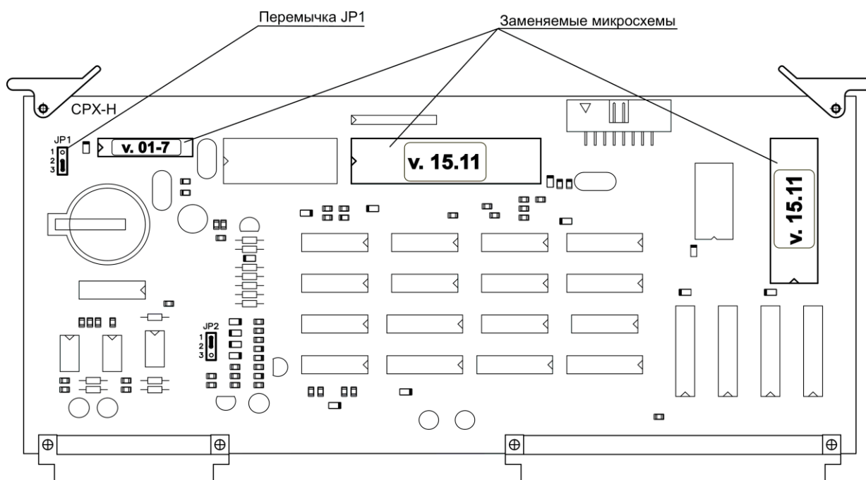
Плата CPX-H
