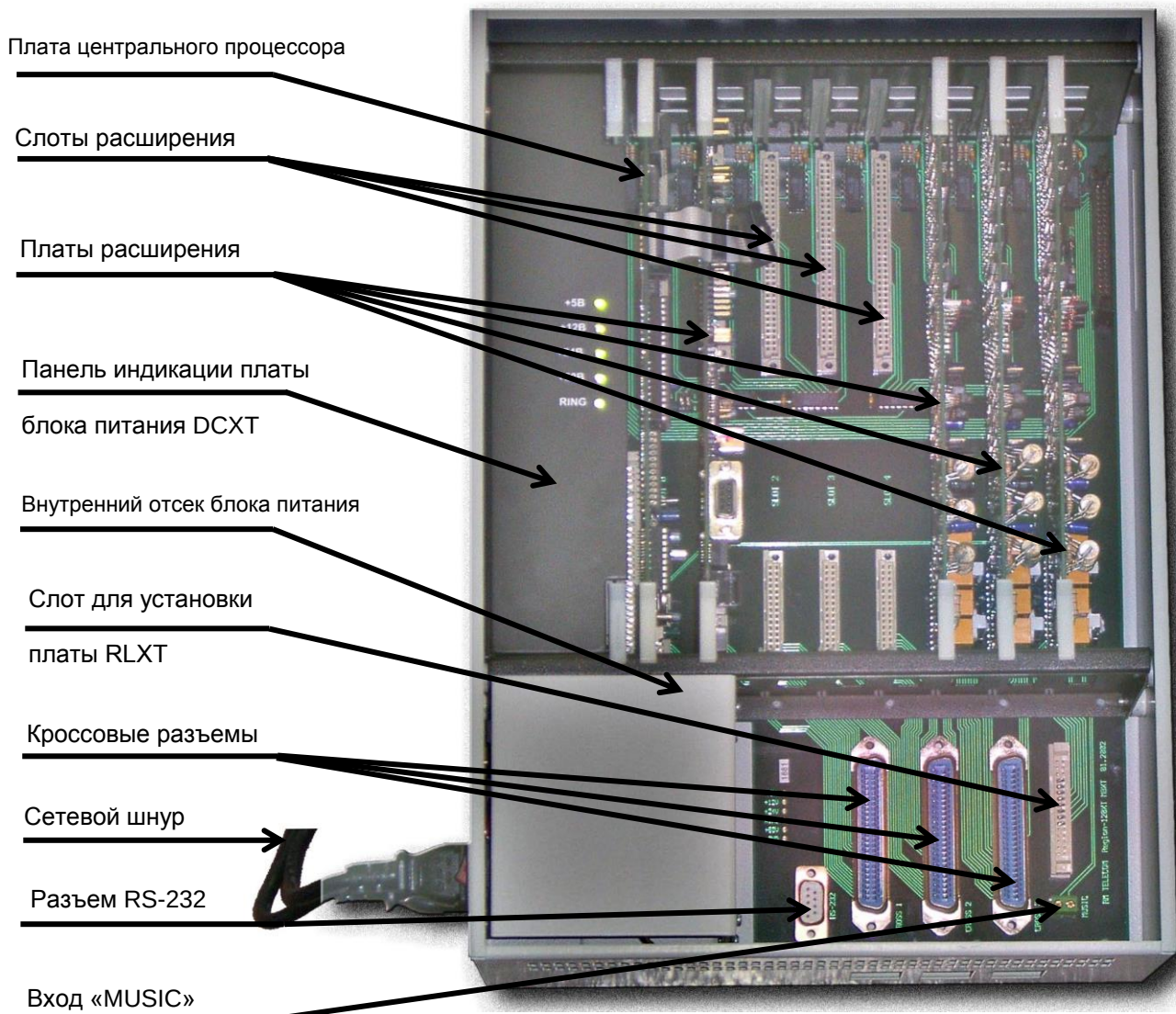
Рис. 1. Базовый блок РЕГИОН-120ХТ.
