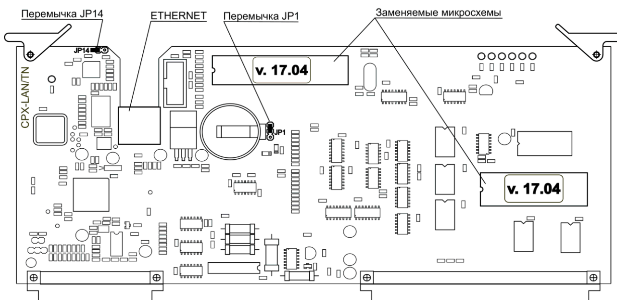
Плата CPX-LAN/TN
