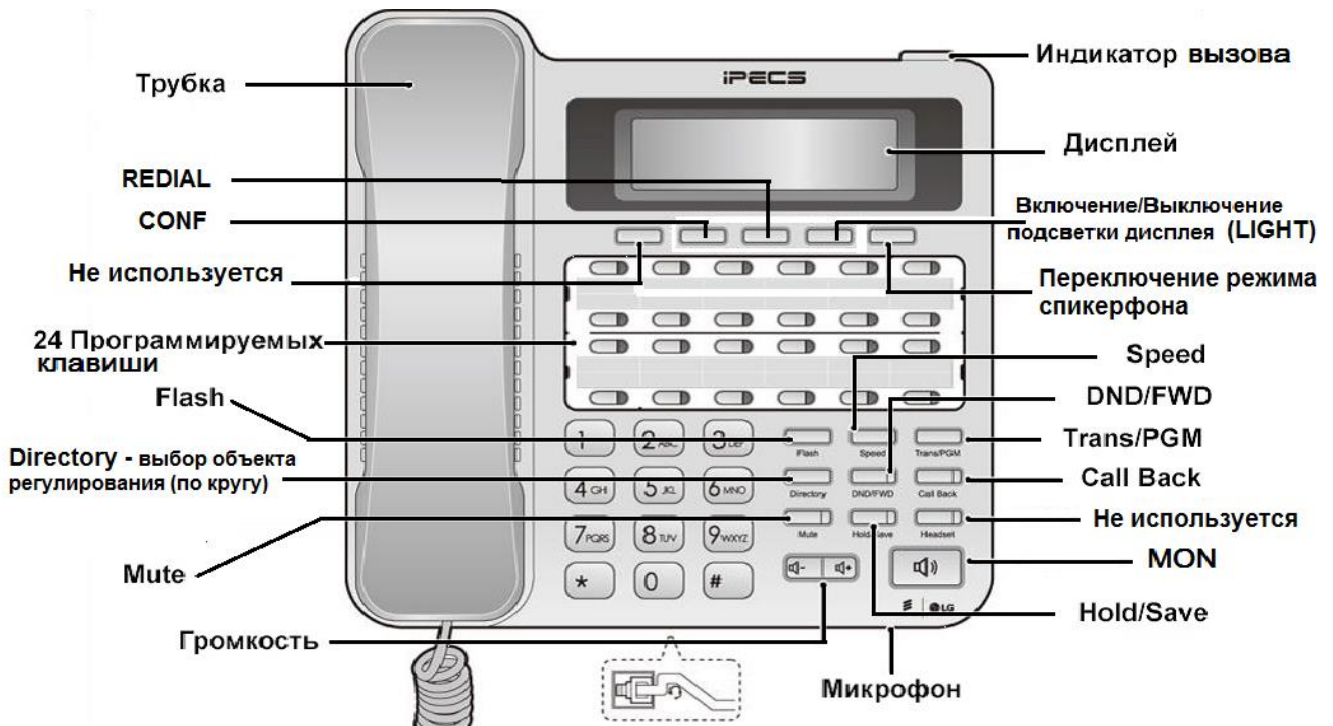
Рис. 7. Расположение клавиш и схема навигации системного аппарата LDP-9224DF
