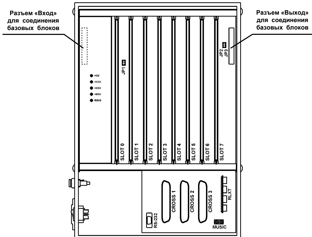
Рис. 2. Нумерация слотов, кроссовых разъемов и перемычек в базовом блоке.
