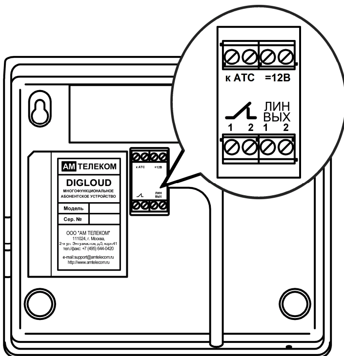
Рис. 4. Расположение клемм для подключения внешних устройств.
