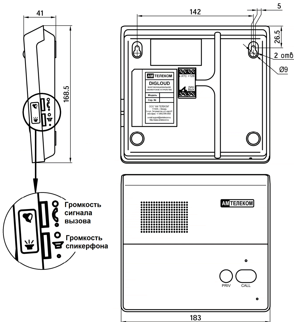
Рис. 1 Внешний вид и габаритные размеры устройства DIGLOUD-B.
