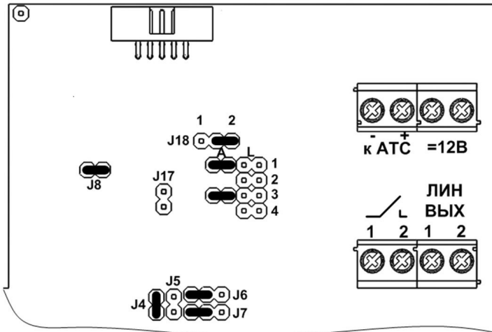
Рис. 3. Схема расположения настроечных перемычек на плате. (указано расположение перемычек при работе с АТС в режиме симплекс, без функции FLASH и с абонентским шлейфом 1 кОм)
