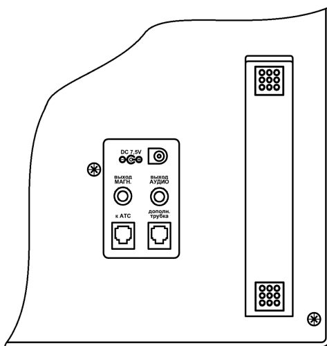
Рис. 2. Разъемы на нижней стороне корпуса РЕГИОН-ЦЛП
