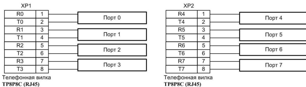
Рис. 24. Схема кабеля для подключения оконечных абонентских устройств
