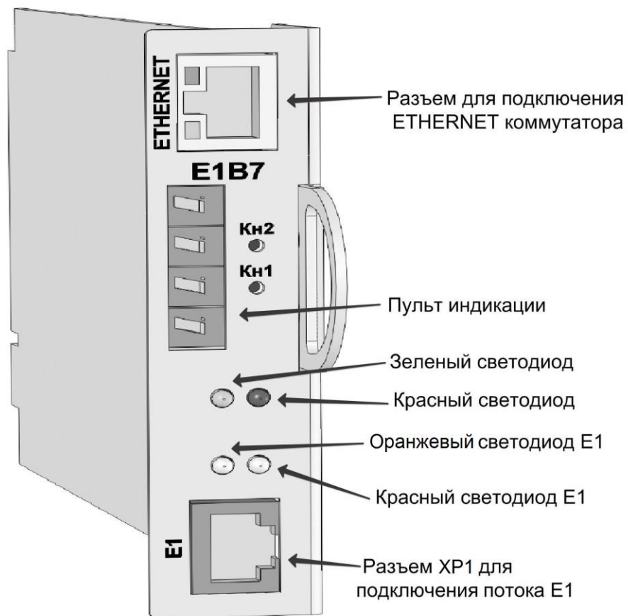
Рис. 15. Модуль E1B7
