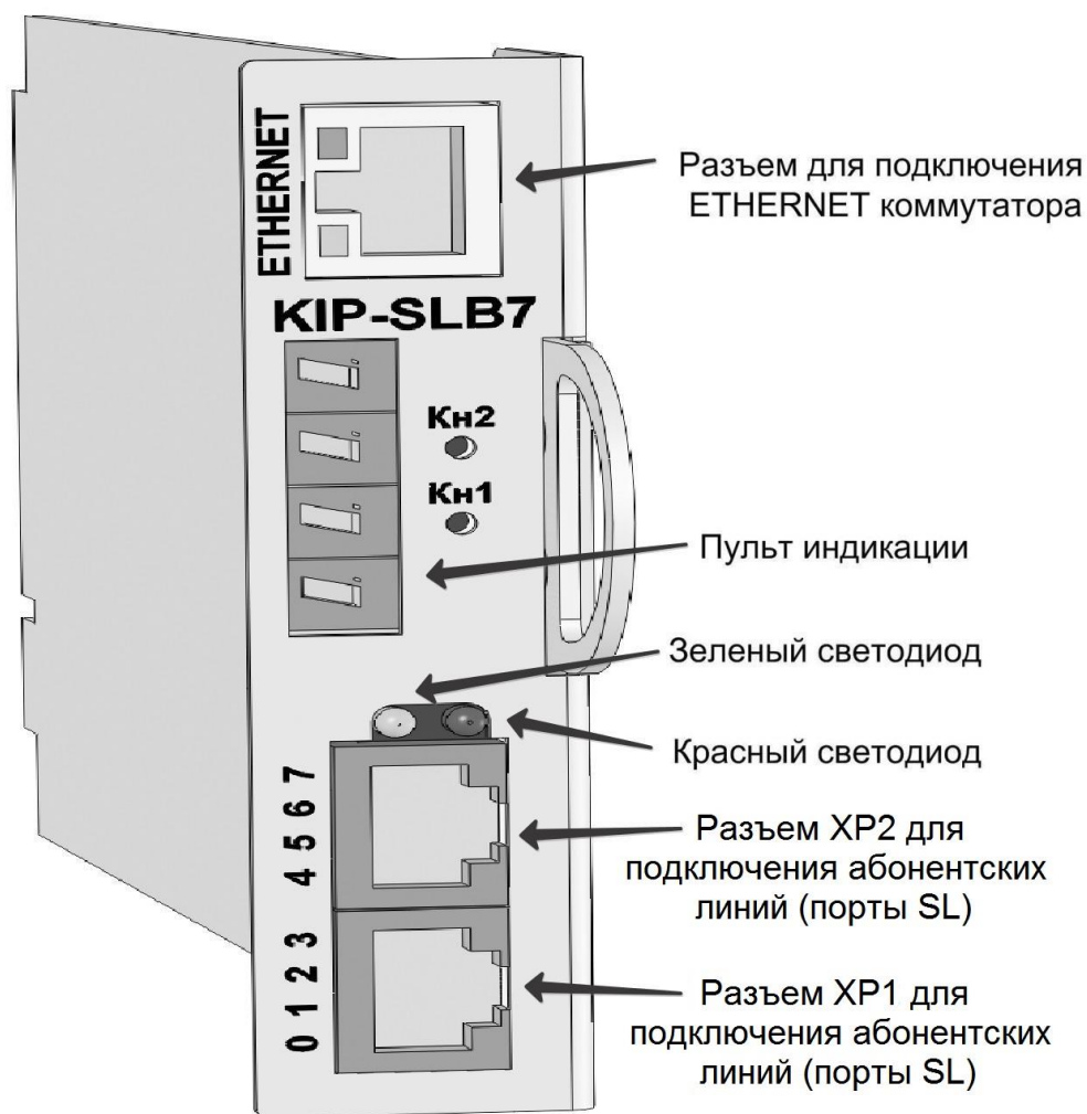
Рис. 22. Модуль KIP-SLB7
