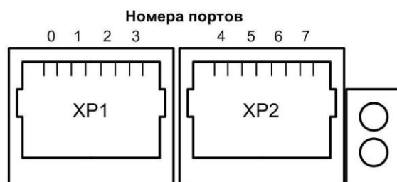
Рис. 3. Разъемы модуля SLB7-08 для подключения абонентских линий
