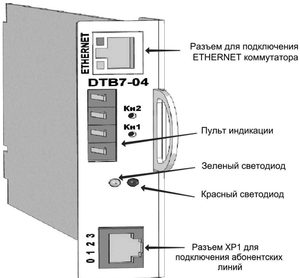
Рис. 28. Модуль DTB7-04
