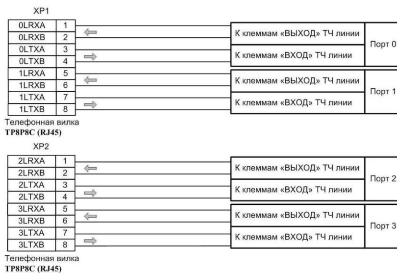
Рис. 27. Схема кабеля для подключения линий
