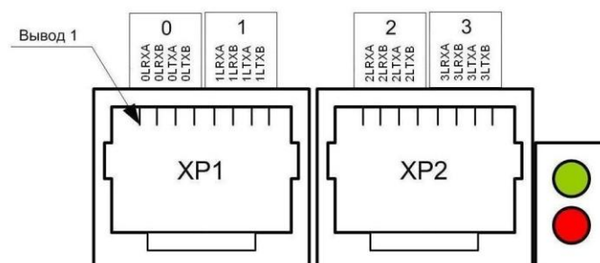
Рис. 26. Разъемы модуля TFB7-04 для подключения абонентских линий
