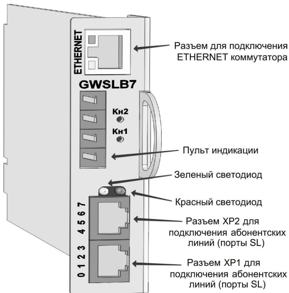
Рис. 19. Модуль GWSLB7
