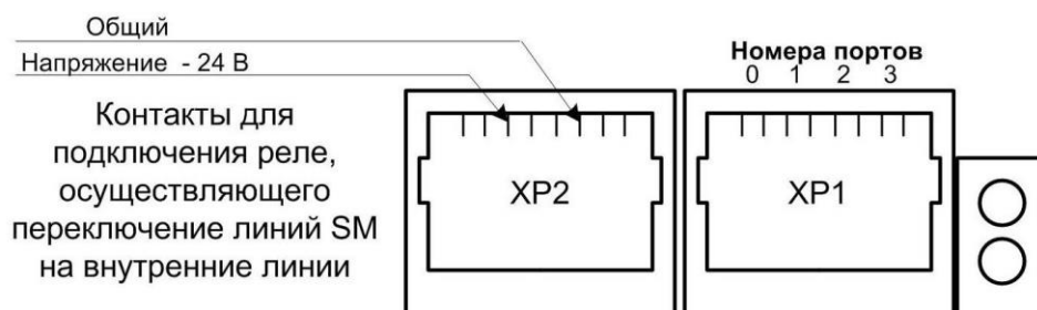
Рис. 9. Разъемы модуля SMB7-04 для подключения линий SM
