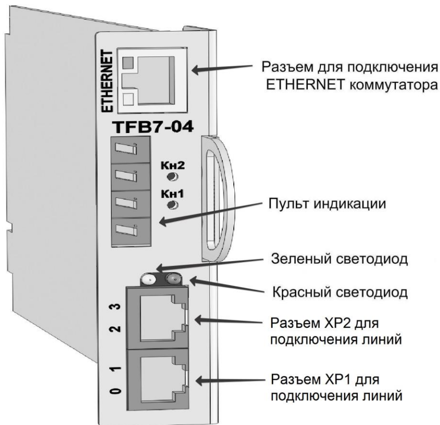
Рис. 25. Модуль TFB7-04
