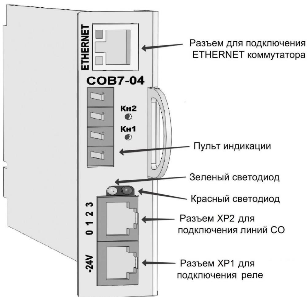
Рис. 5. Модуль COB7-04
