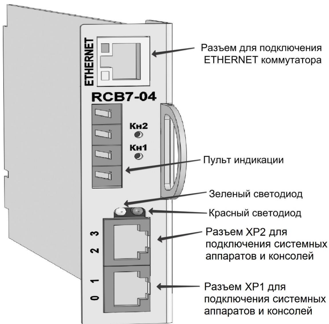
Рис. 12. Модуль RCB7-04
