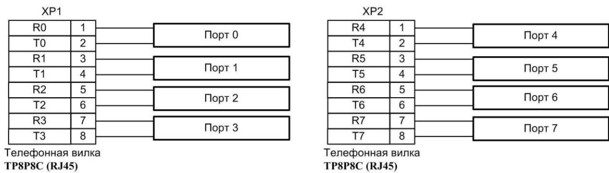
Рис. 4. Схема кабеля для подключения оконечных абонентских устройств
