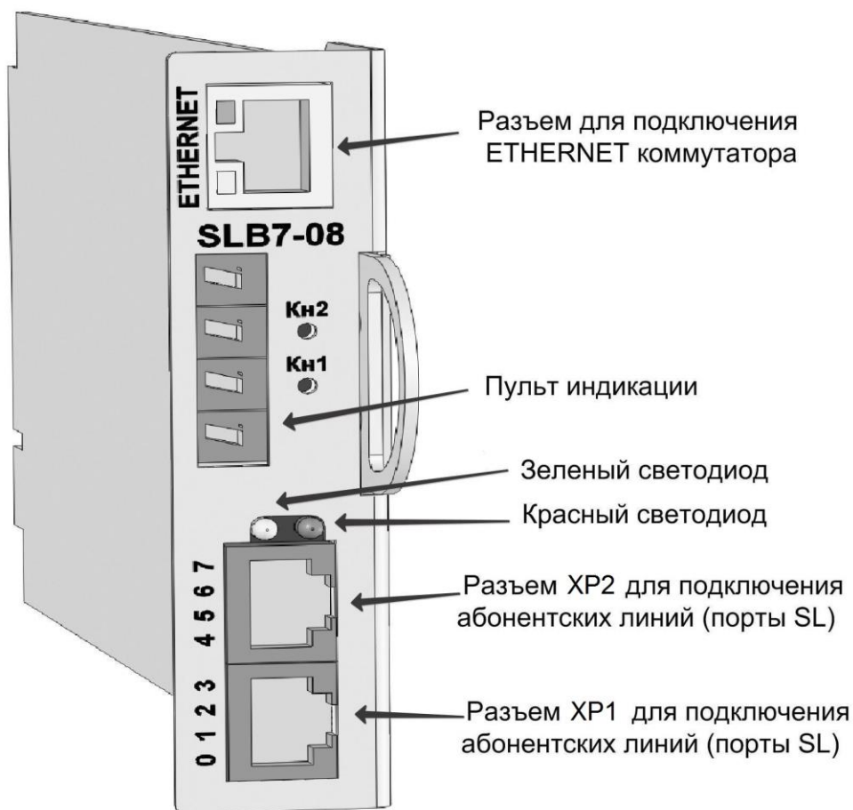
Рис. 2. Модуль SLB7-08
