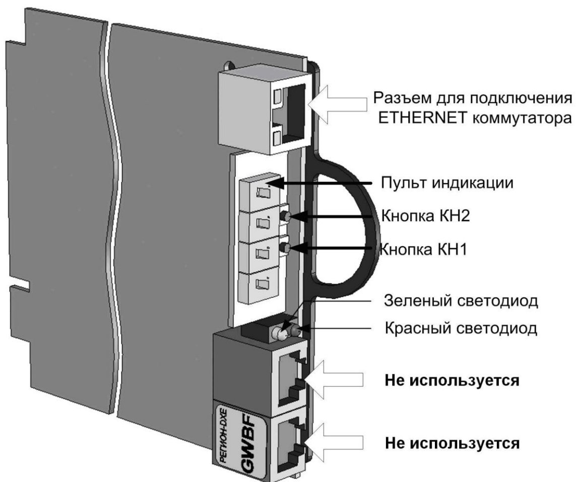
Рис. 18. Модуль GWBF
