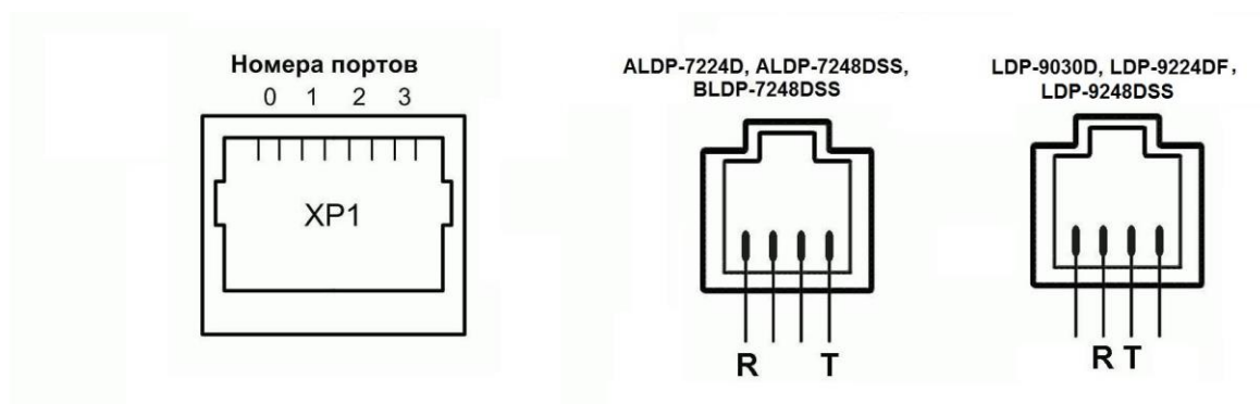
Рис. 29. Разъем модуля DTB7-04, системных аппаратов и консолей для подключения абонентских линий
